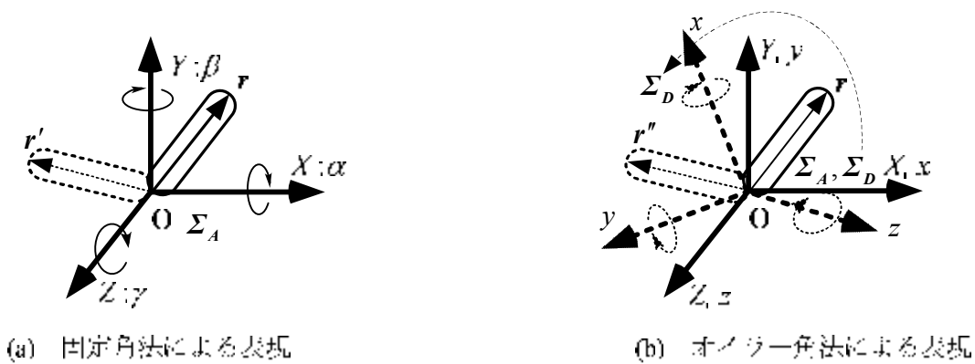
図4.15 姿勢表現の方法と比較
