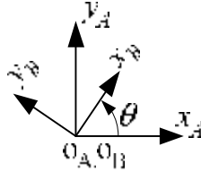
図 4.4 回転行列による姿勢の表現
