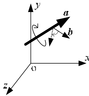
(b) 有顔ベクトルによる姿勢の表現
