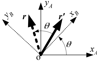
図 4.5 姿勢変化表現のための回転演算子
