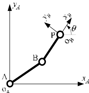
図 4.3 回転行列を利用した平面における位置・姿勢表現*1（ここではベースと出力リンク上のみ座標系を設定し説明する．各ジョイント上に設定するのは後述）
