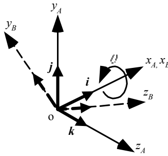
図 4.8 X 軸まわりの回転行列
